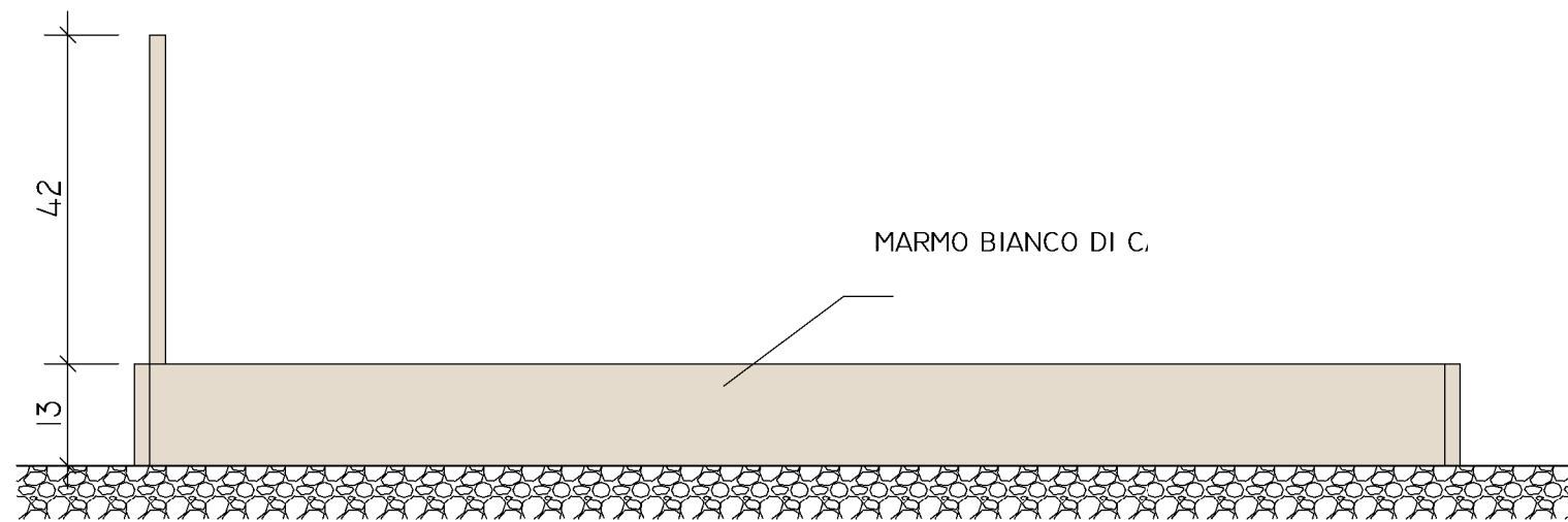
PROSPETTO LATERALE SCALA 1/10
