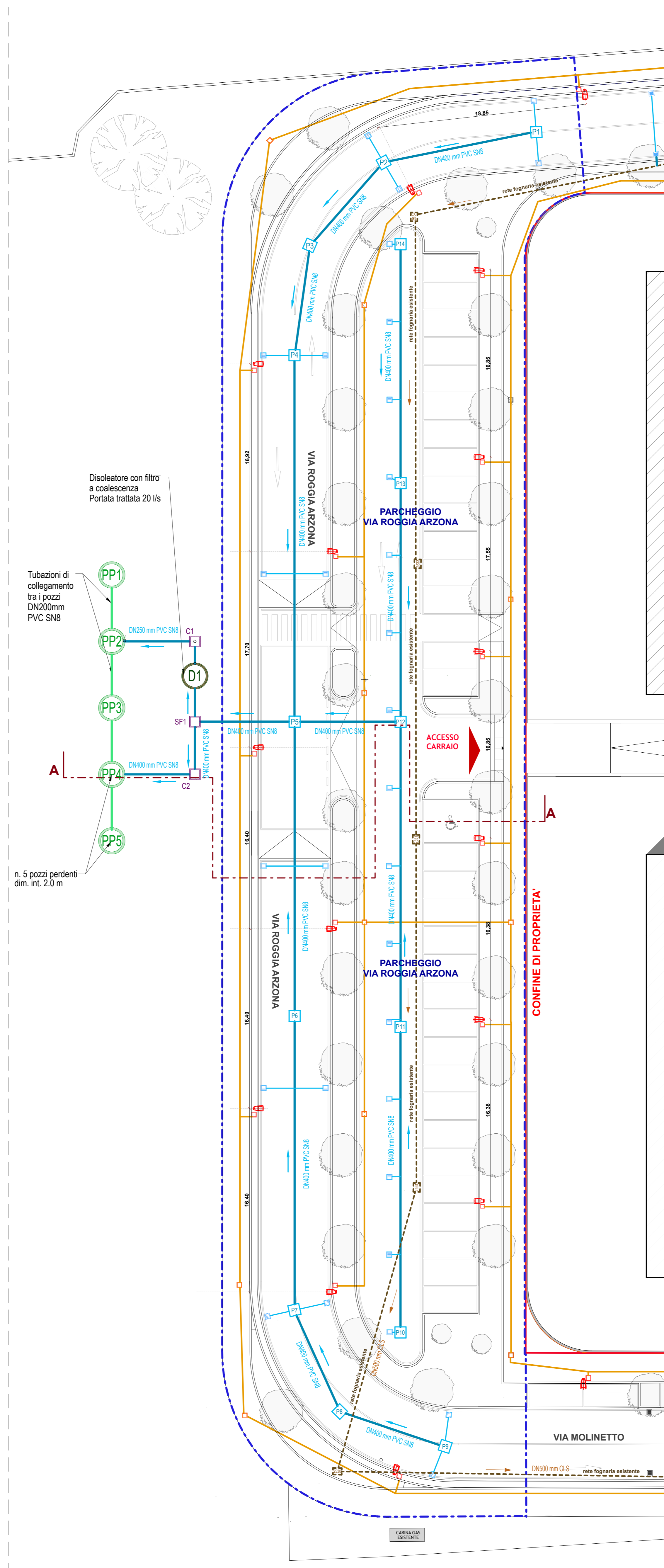
PLANIMETRIA IMPIANTI
