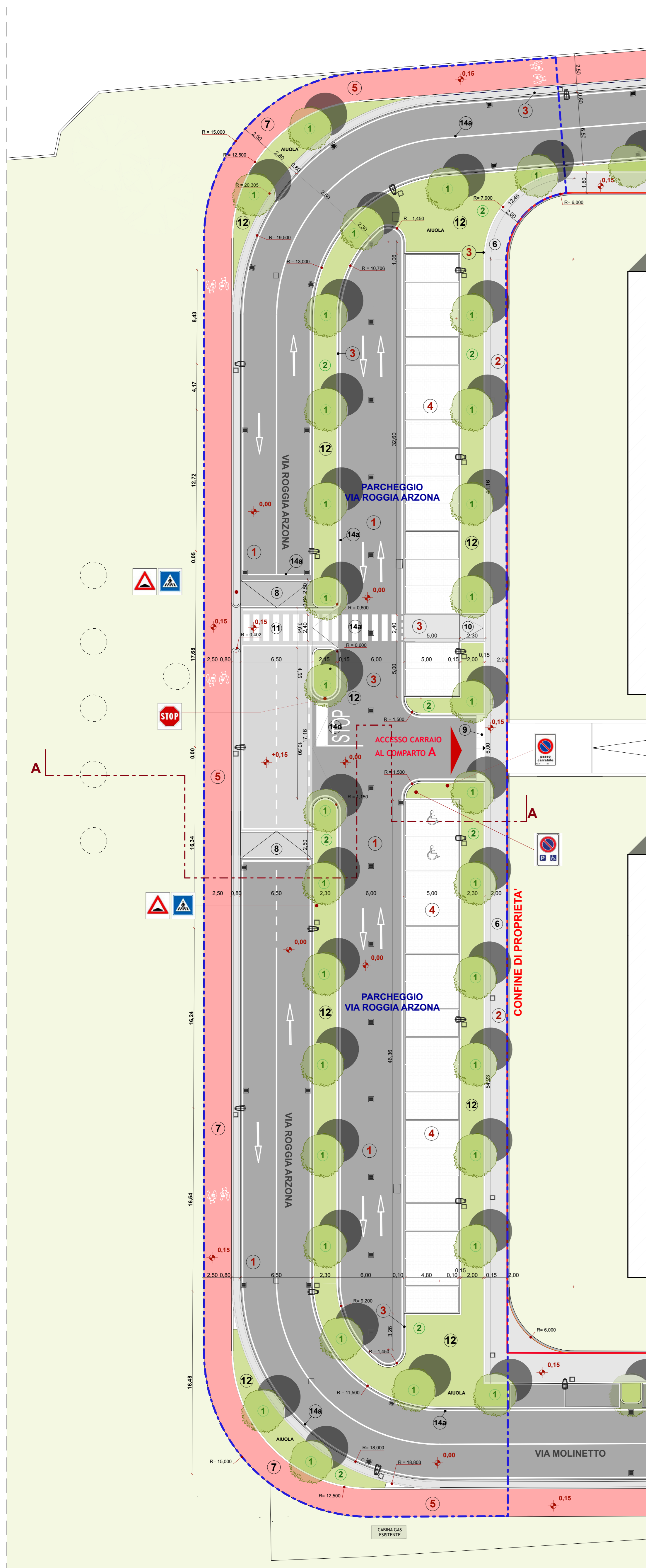
PLANIMETRIA GENERALE - MATERIALI
