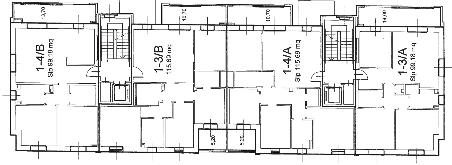
PIANO PRIMO
