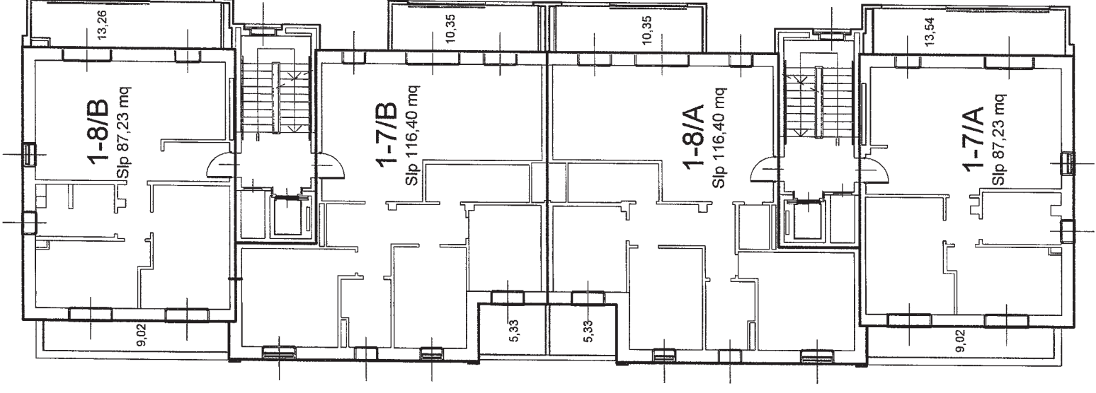
PIANO TERZO
