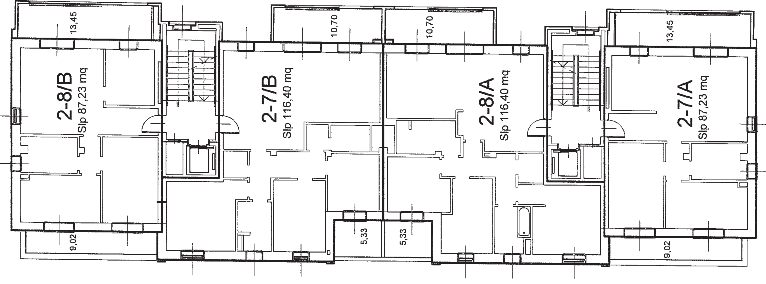
PIANO TERZO
