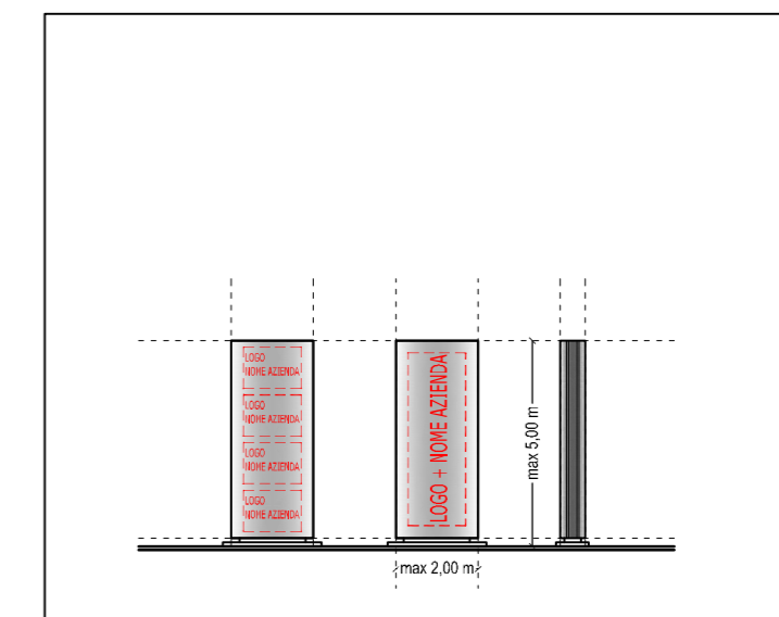
SCHEMA TOTEM PUBBLICITARIO
