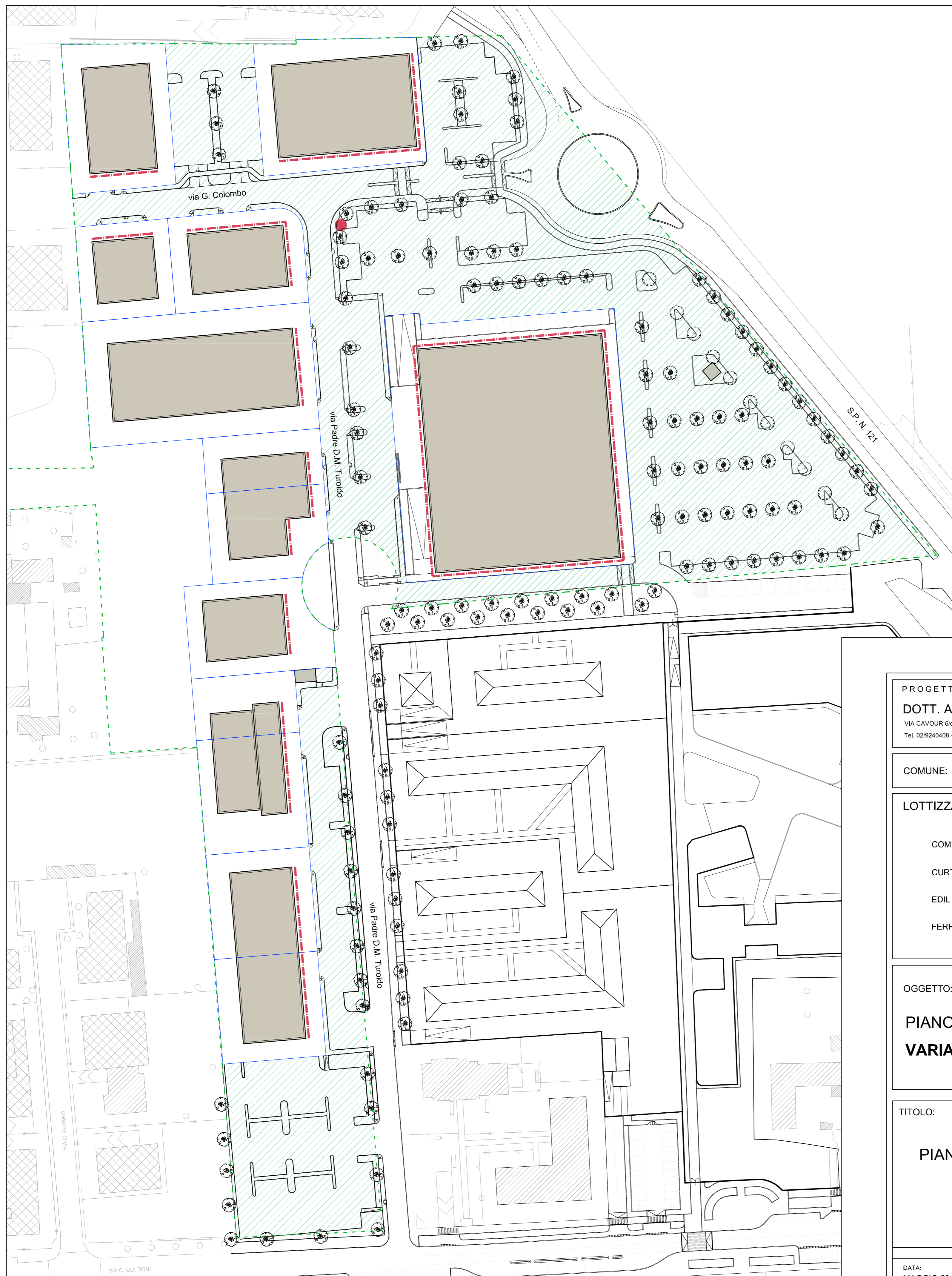
PLANIMETRIA GENERALE SCALA 1:750
