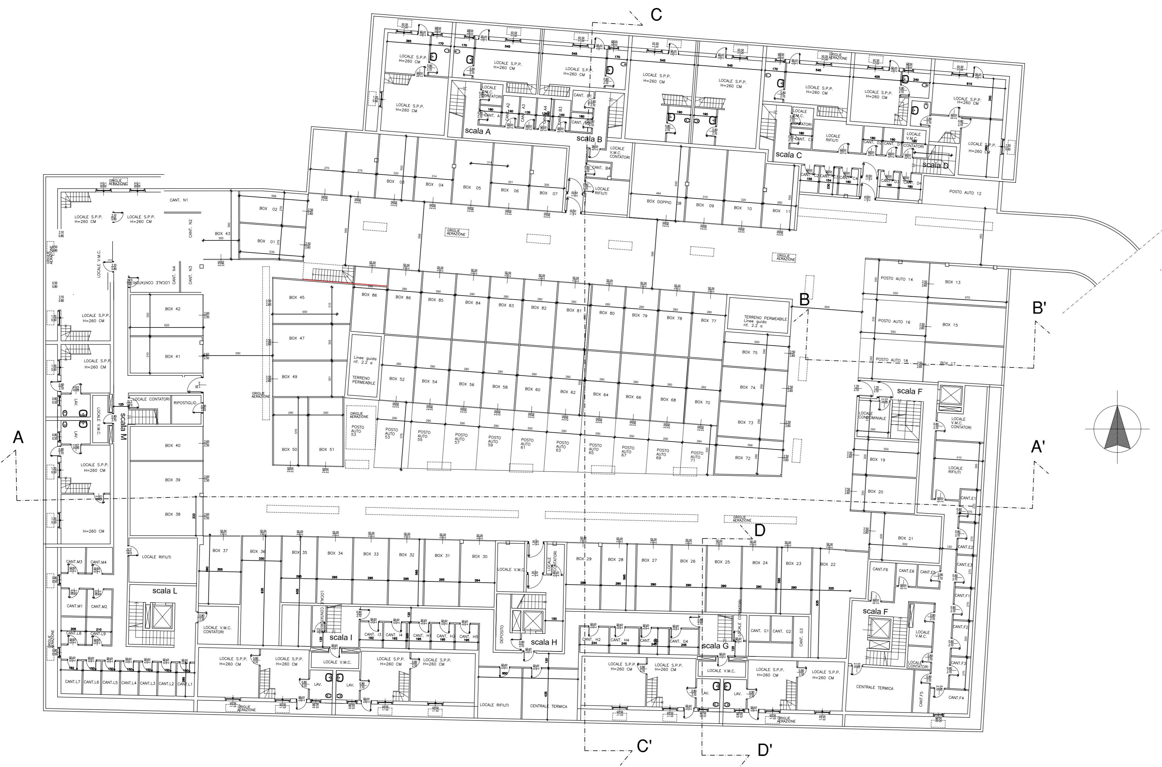
Pianta Piano Interrato
