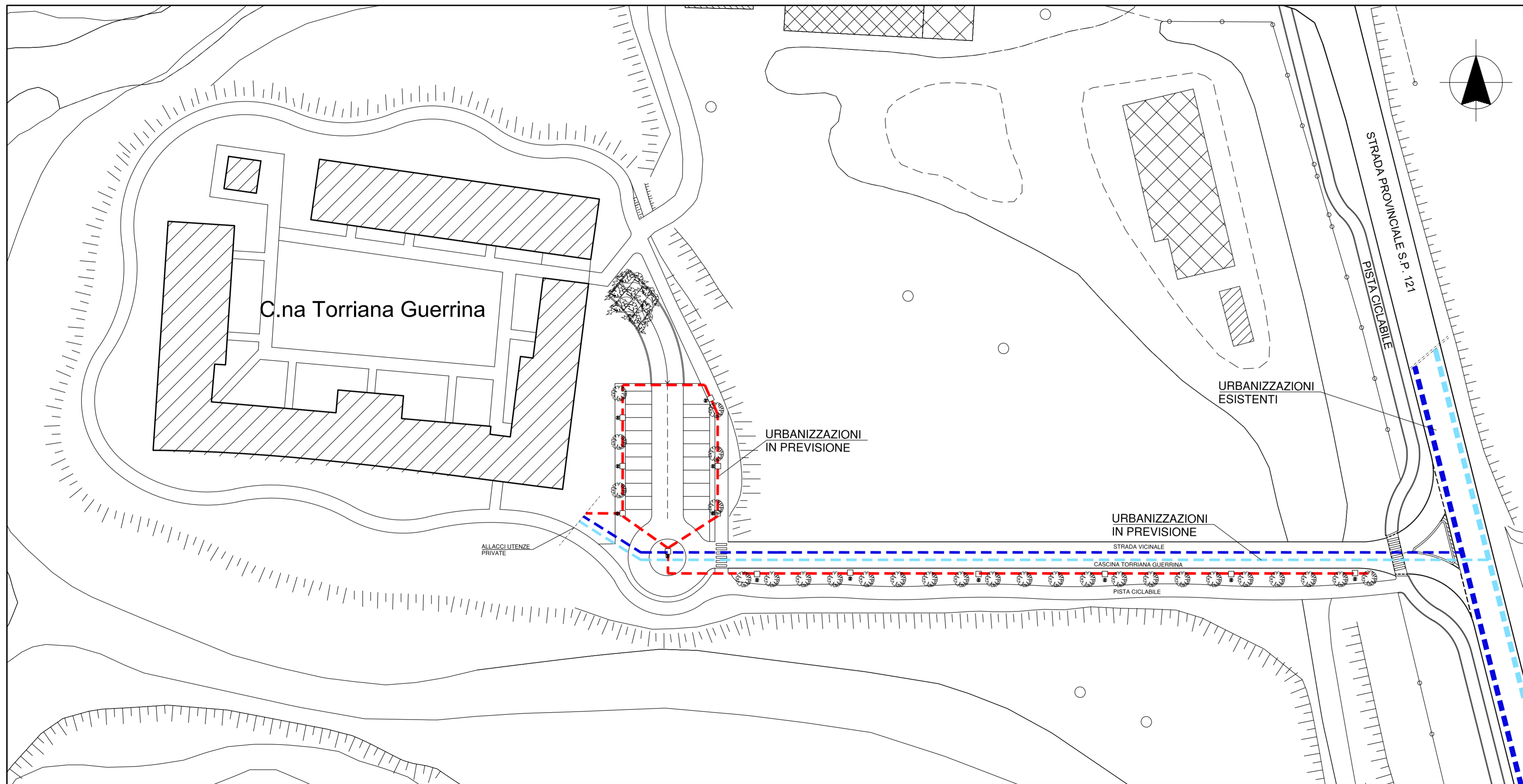
SCHEMA RETE SERVIZI TECNOLOGICI
